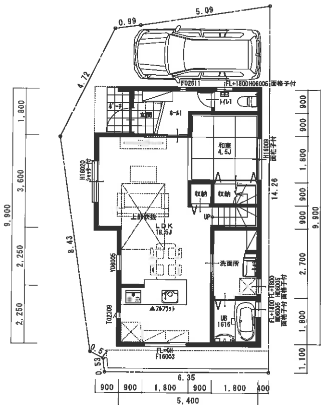
1階 平面図 S=1/100
