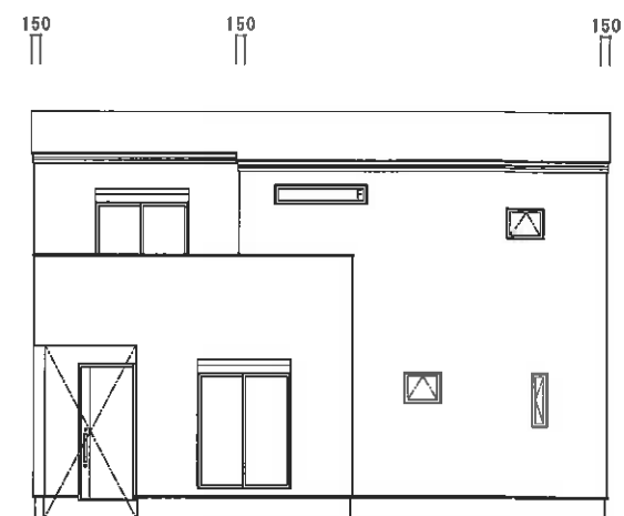
西側立面図
