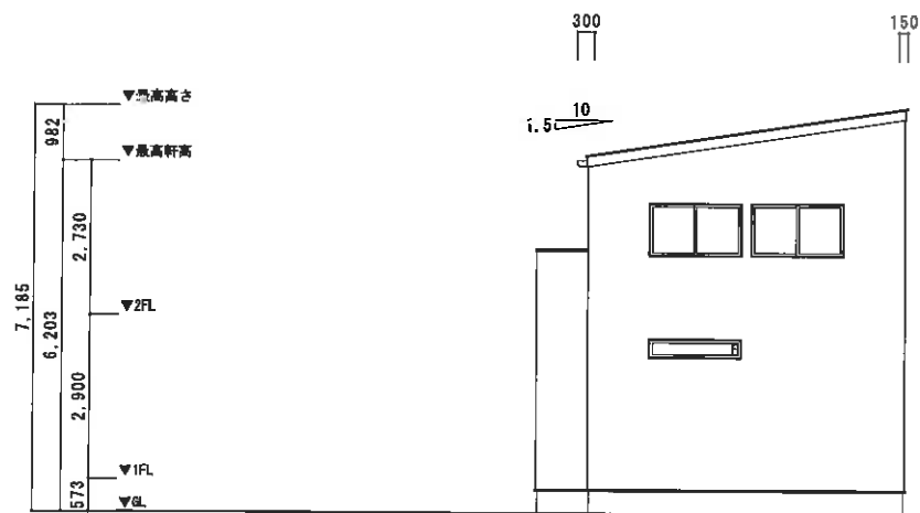
南側立面図
